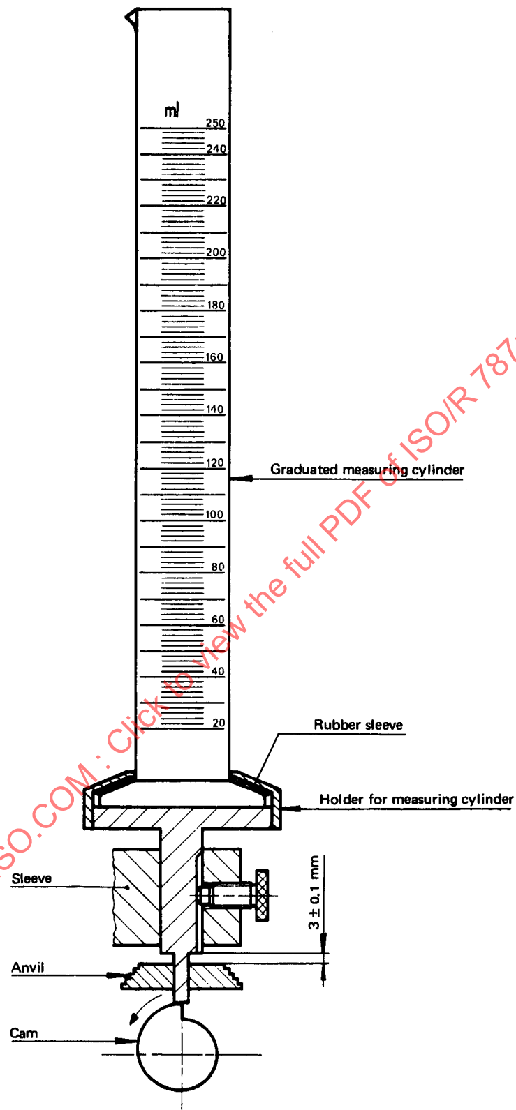
FIG. 2 — Tamping volumeter
