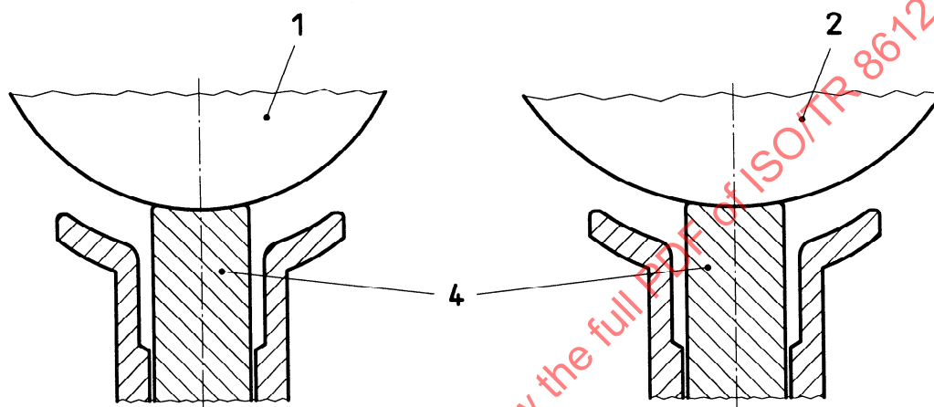
b) Plunger
