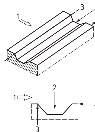
f) Ditch
