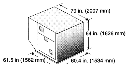
Type : LD-3 container / IATA - AKE
