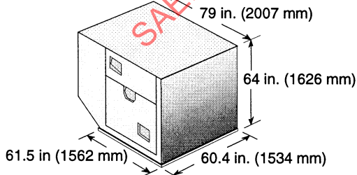
Type : LD-3 container / IATA - AKE
