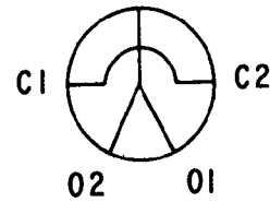
Edgetone
