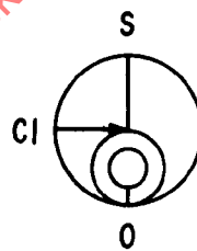
Vortex
