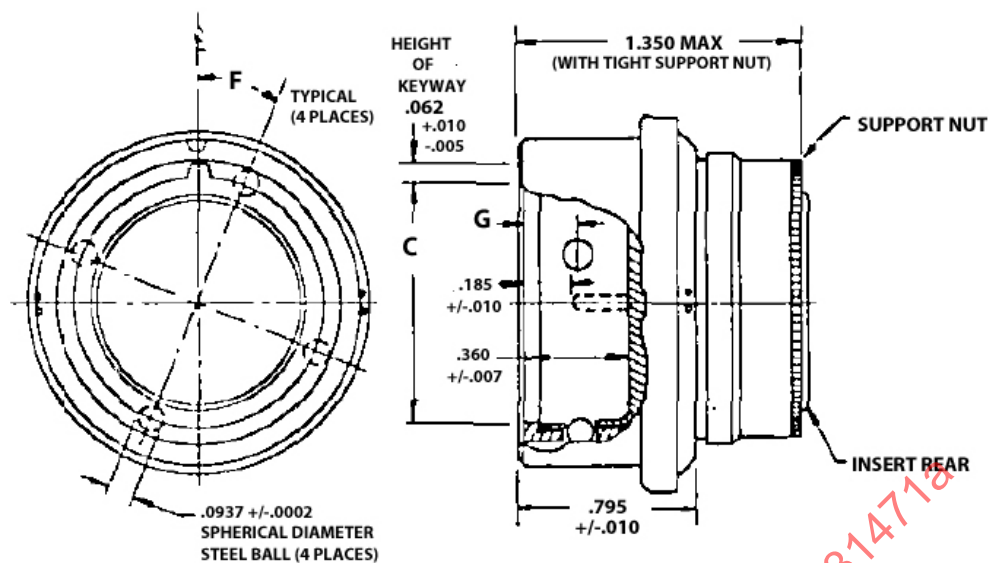
STYLE P (PIN INSERT)
