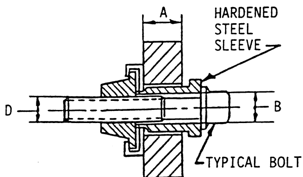
FIGURE D1 - Torque Out Test Apparatus
