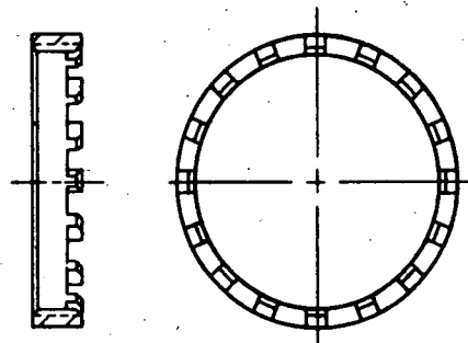
Spanner nut
