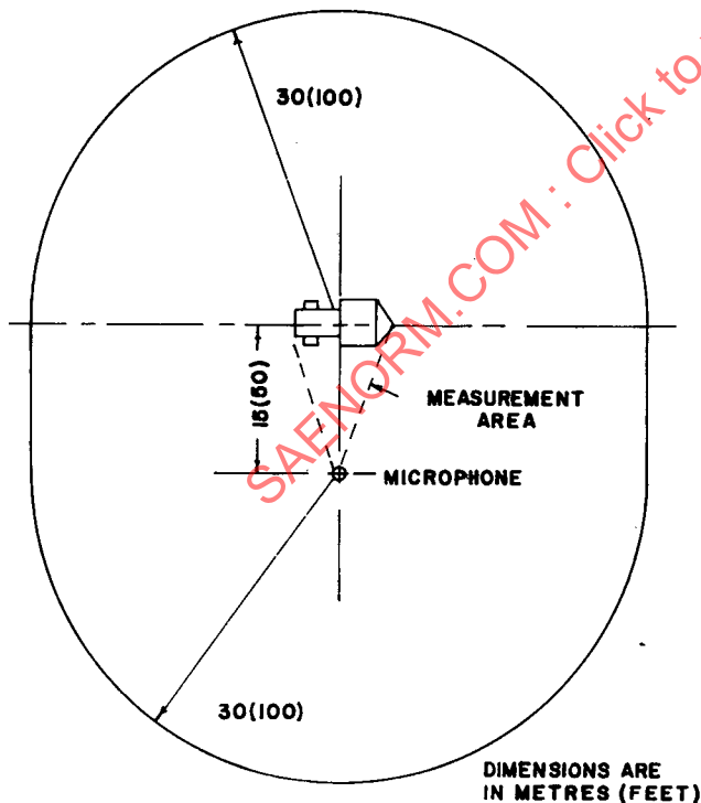
FIG. 1—TEST SITE CONFIGURATION
