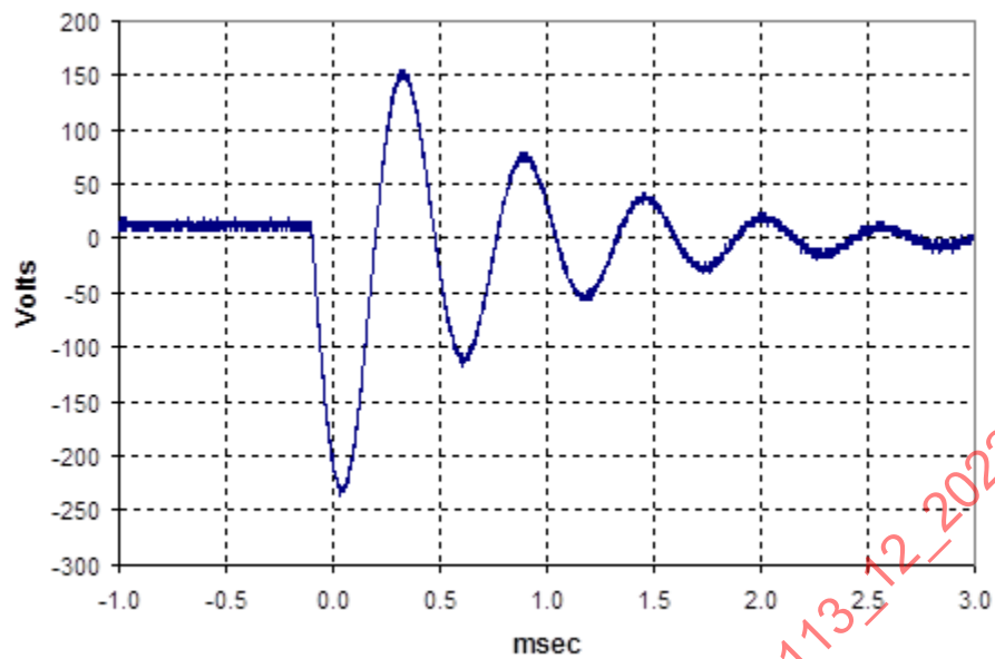
b) Pulse B1
