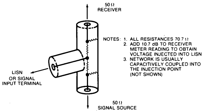
FIG. 5(A) - Z_G = Z_R = 50 \Omega
