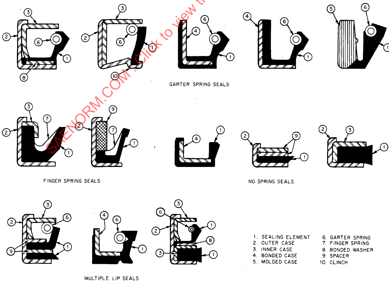
FIG. 3—COMPONENTS
