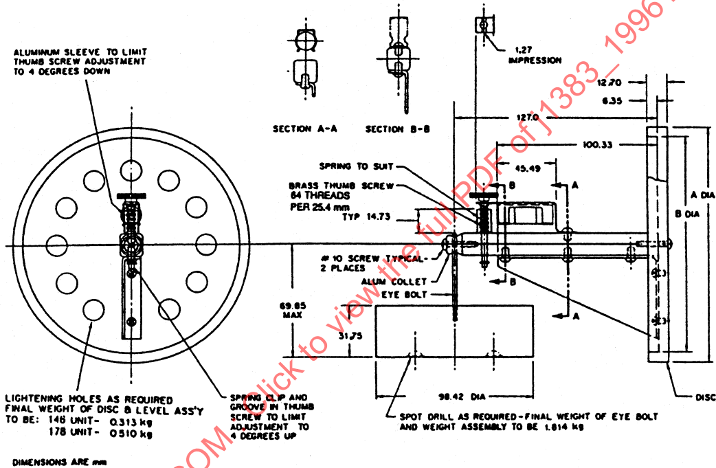
FIGURE 4—DEFLECTOMETER
