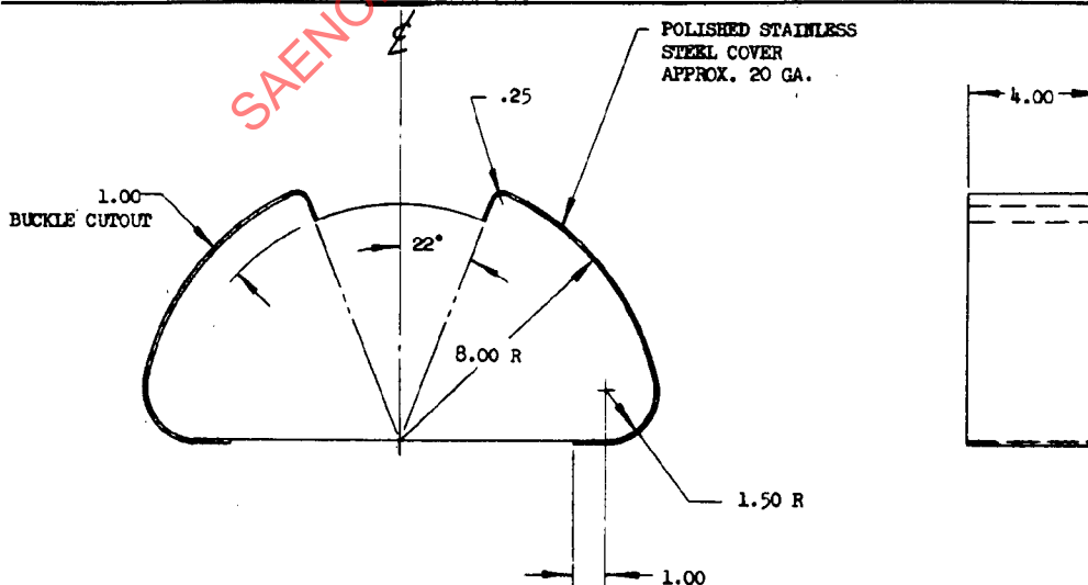
Fig. 1 - Abrasion test
