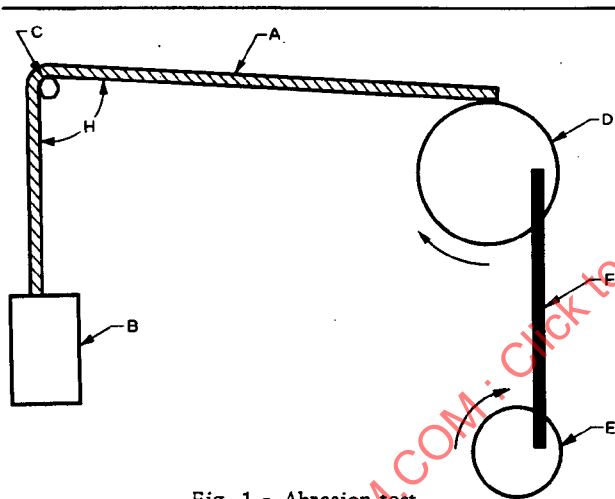
Fig. 1 - Abrasion test
