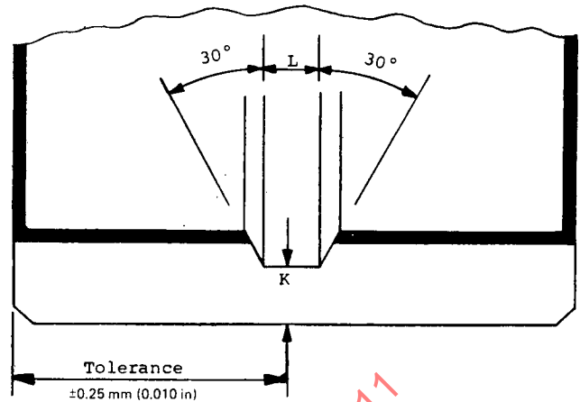
FIG. 9—GROOVE DIMENSIONS
