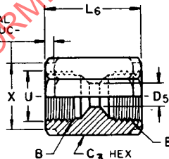
FIG. 8—INTERNAL FLARE UNION (010107) (U4)
