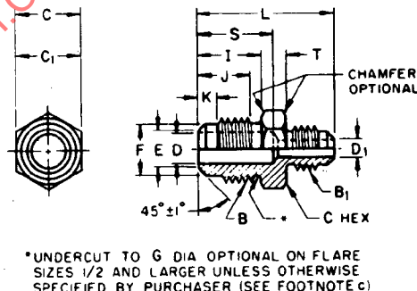
FIG. 21—REDUCING UNION (010101) (UR2)
