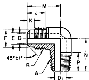
FIG. 11—90 DEG ELBOW (010202) (E1)
