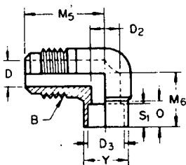
FIG. 16—90 DEG SOLDER ELBOW (010204) (ES)
