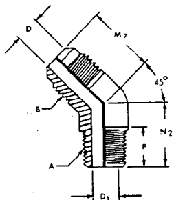
FIG. 13—45 DEG ELBOW (010302) (E5)
