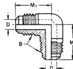
FIG. 12—90 DEG ELBOW UNION (010201) (E2)
