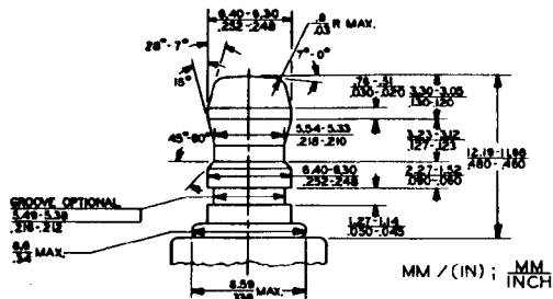
FIG. 7—SOLID POST TYPE
