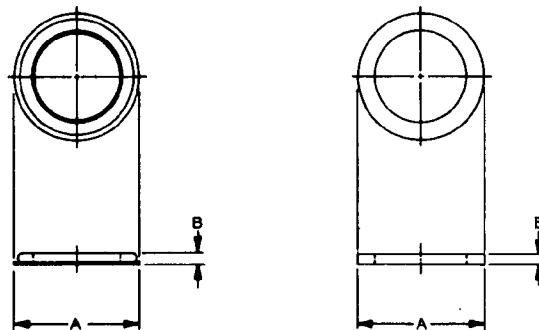
FIG. 6—GASKETS (SEE TABLE 5)
