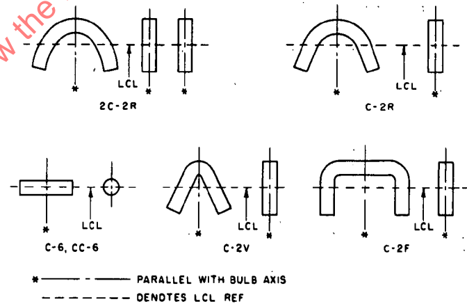
FIG. 4—FILAMENT TYPES
