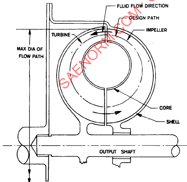
FIG. 1—FLUID COUPLING
