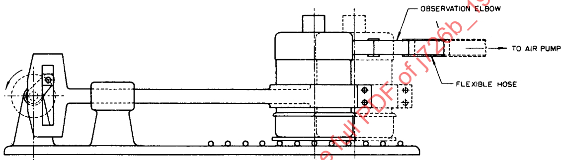
FIG. 7B—HORIZONTAL SHAKE
