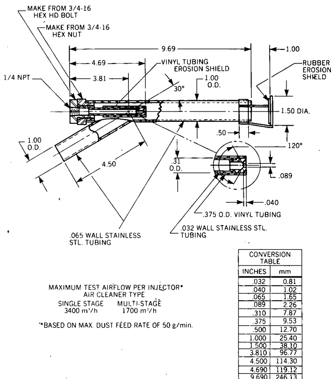
FIG. 3F—DUST INJECTOR
