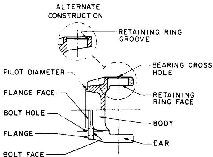
FIG. 6—FLANGE YOKE
