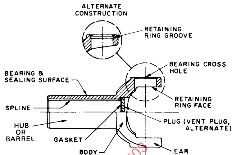
FIG. 2—SLIP YOKE
