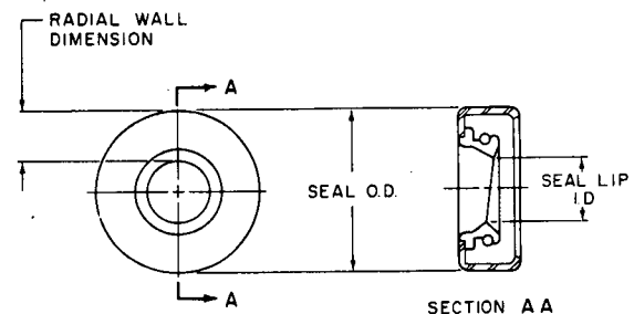
FIG. 6—RADIAL WALL DIMENSION
