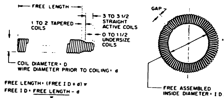
FIG. 10 - SPRING NOMENCLATURE
