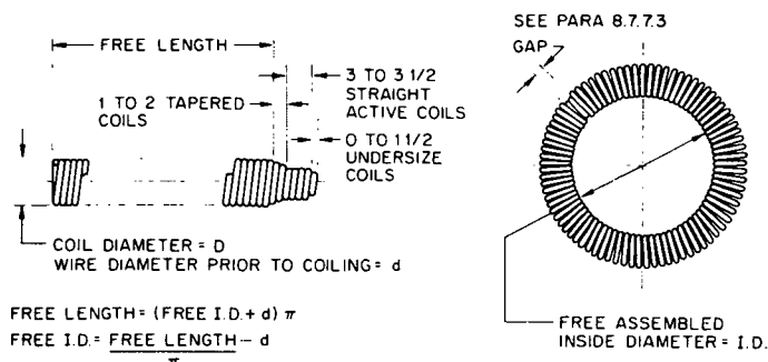
FIG. 14—SPRING NOMENCLATURE
