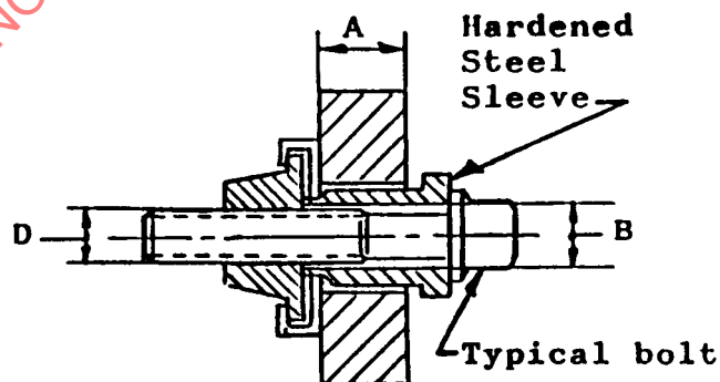
FIGURE D1 - Torque Out Test Apparatus
