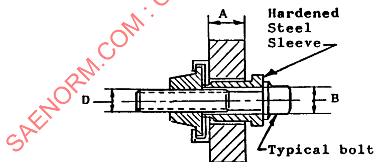
FIGURE D1 - TORQUE OUT TEST APPARATUS
